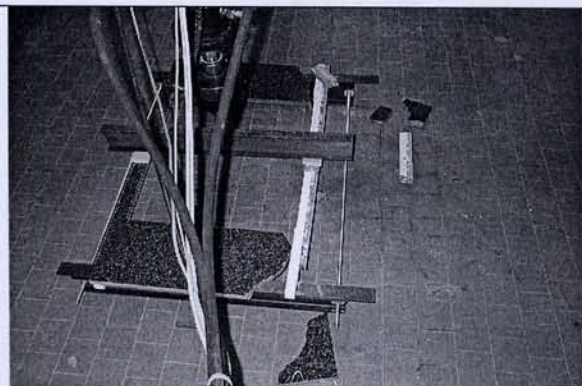
Bild 3: Probekörper 2
